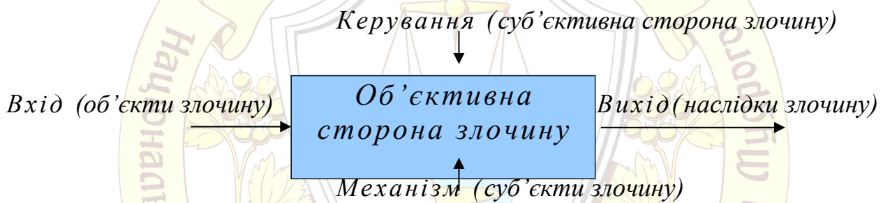
Рисунок. IDEF0-модель злочину
